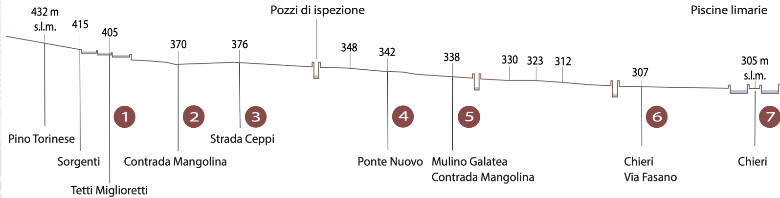
Sezione altimetrica dell'acquedotto con vasche limarie
