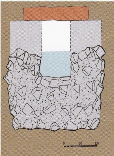
Sezione dell'acquedotto
